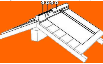
Állókorcos fémlemezfedés gerinc kiszellőzésének csomóponti ábrája
